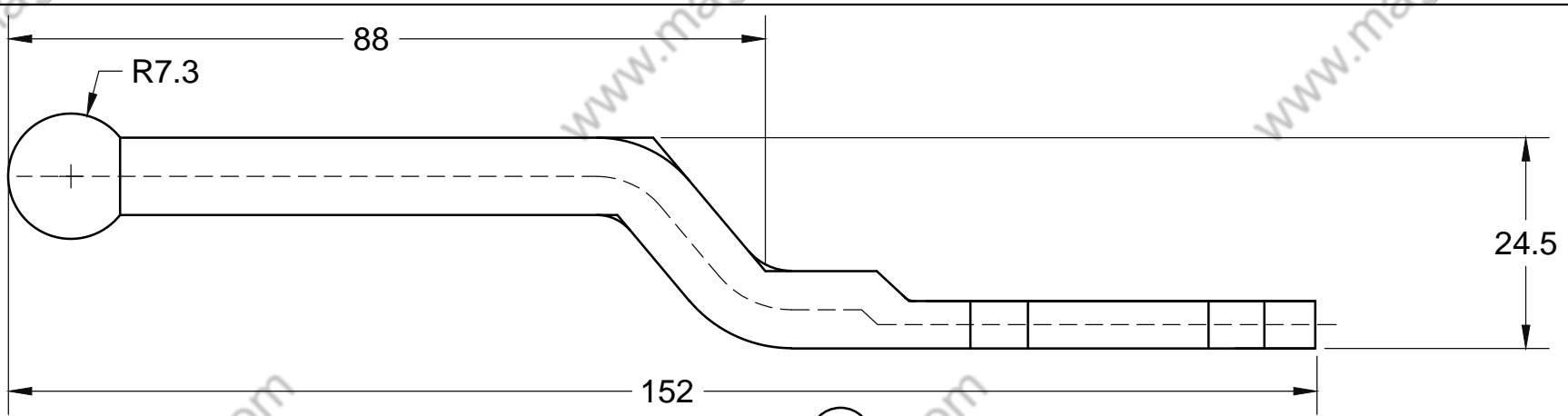
② ROD HANDLE
